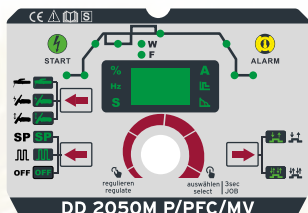
Upravljalna plošča DD 2050M P/PFC/MV
