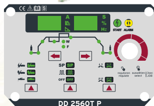
Upravljalna plošča DD 2560T P
